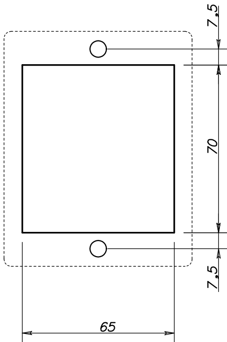
DIMENSIONI SCASSO
